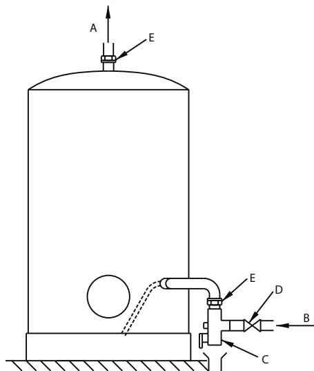
Abbildung 12 - Geräte auf Sockel
