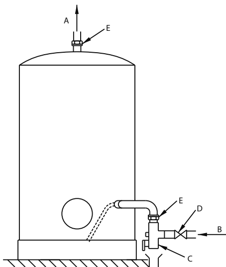
Afbeelding 12 – Model op voetstuk
